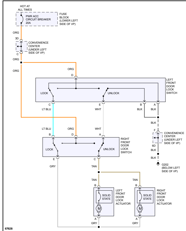
Fig 1: Door Lock Circuit, 2 Door
