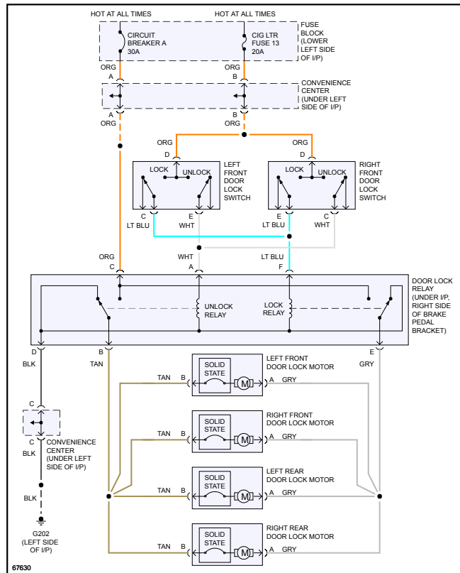
Fig 2: Door Lock Circuit, 4 Door
